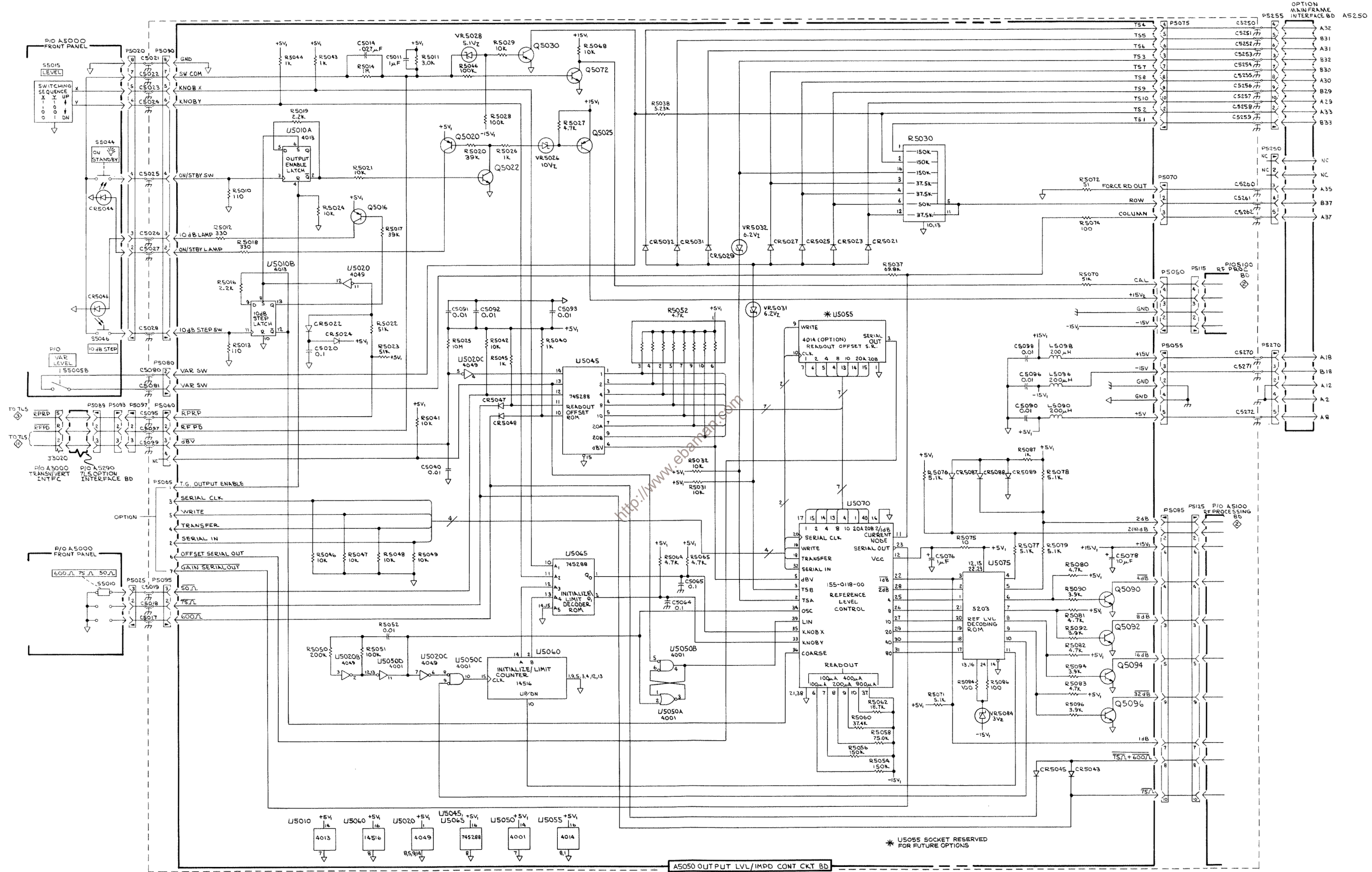
AS250 OUTPUT LVL/IMPED CONT CKT BD
